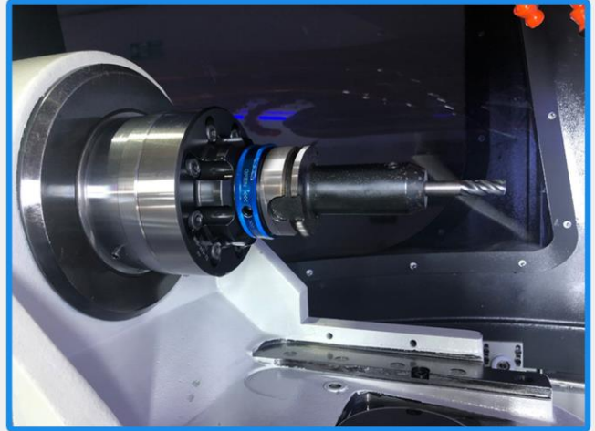
HSK - A63 Takım Tutucu
