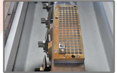
Fixation magnétique pour inserts remplaçable optionnel
